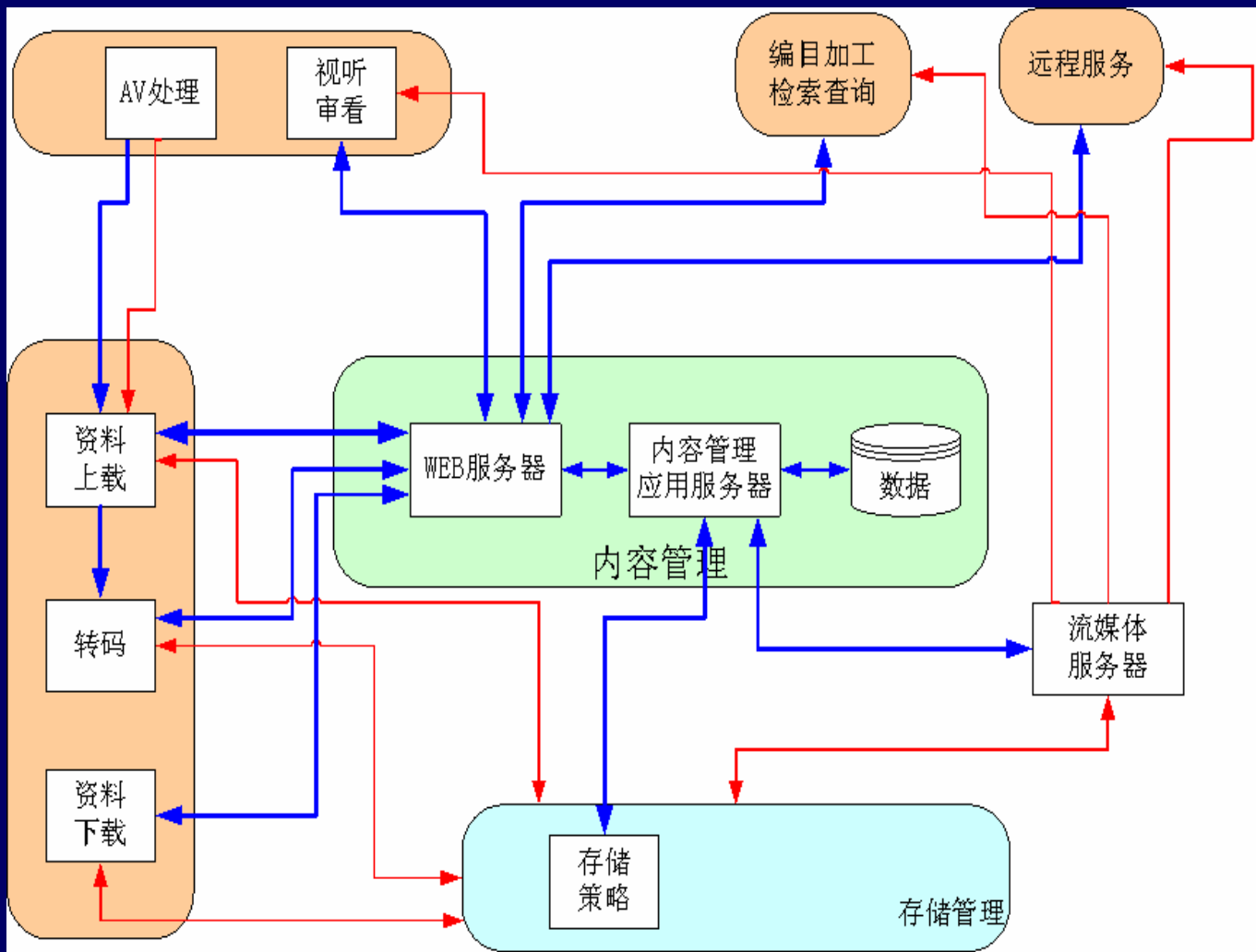
音像资料馆系统逻辑图
